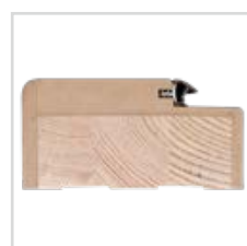
Fix ajtótok fa RC2-ben vagy megerősített RC3-ban
