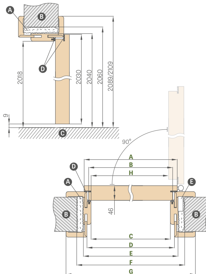
HERSE SET ÁLLÍTHATÓ AJTÓTOK SÉMA
