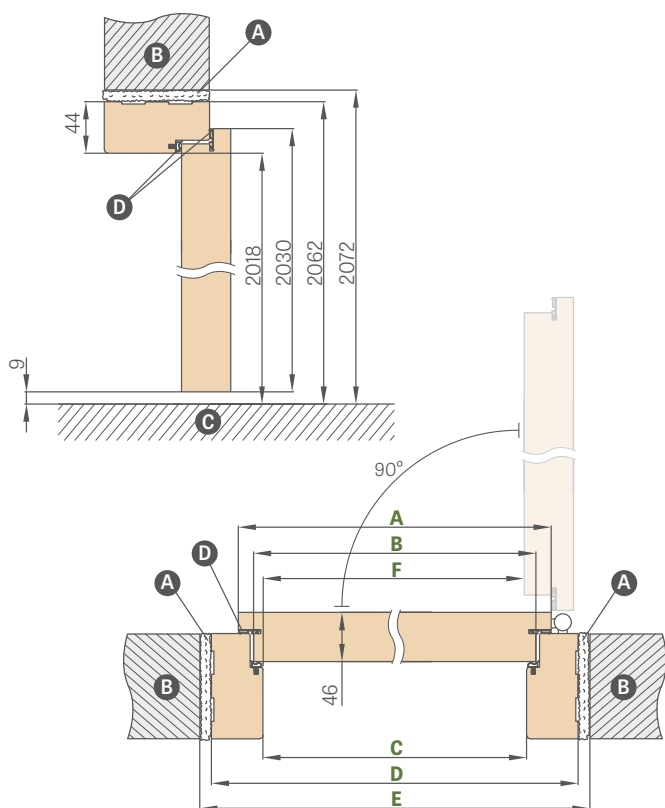
HERSE SET FIX AJTÓTOK SÉMA
