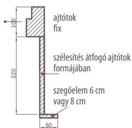
ajtótok bővítése
